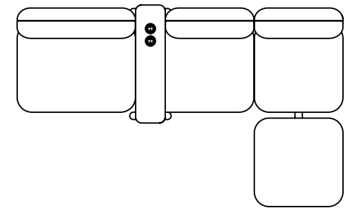
Módulo 80+80+60+60 con 2 respaldos 60+1 respaldo 80 y mesa autoportante 60 80+80+80+60+60 module with 2 backrests 60+1 backrest 80 and self-supporting table 60
