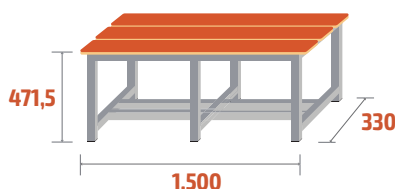
BANC-1-1500 COD: 79001 14kg · 0,23m 3
