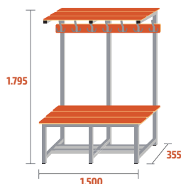
BANC-3-1500 COD: 79023 28,5kg · 0,36m 3 · 7 ↓
