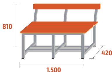
BANC-4-1500 COD: 79325 16,5kg · 0,51m 3
