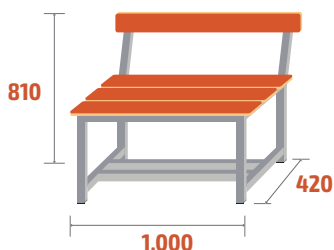
BANC-4-1000 COD: 79300 11,5kg · 0,34m 3
