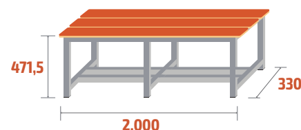
BANC-1-2000 COD: 79020 18kg · 0,31m 3
