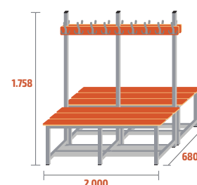
BANC-2-2000-DC COD: 79214 52kg · 0,62m 3 · 18 ↓
