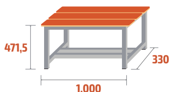
BANC-1-1000 COD: 79010 9,5kg · 0,16m 3
