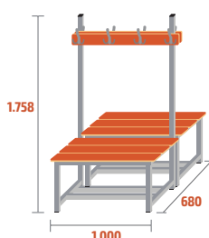
BANC-2-1000-DC COD: 79212 28kg · 0,46m 3 · 8 ↓
