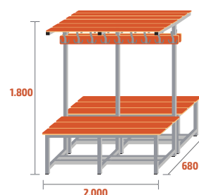
BANC-3-2000-DC COD: 79224 61kg · 0,64m 3 · 18 ↓
