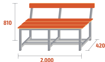
BANC-4-2000 COD: 79350 20,5kg · 0,68m 3
