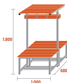
BANC-3-1000-DC COD: 79222 37kg · 0,48m 3 · 8 ↓
