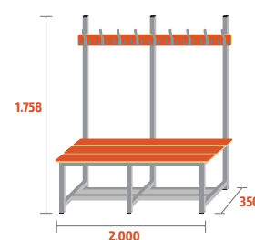
BANC-2-2000 COD: 79014 29kg · 0,31m 3 · 9 ↓
