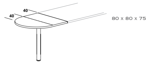
EXTENSIÓN SEMICIRCULAR. SEMICIRCULAR EXTENSION. LIAISON DEMI-RONDE.
